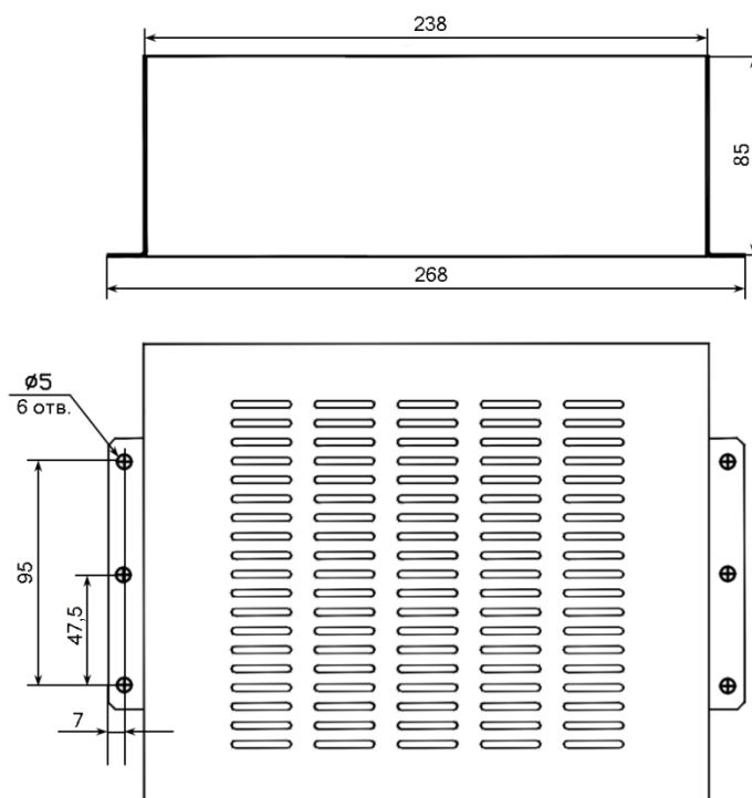
Рисунок 1 - Габаритные размеры защитного кожуха
